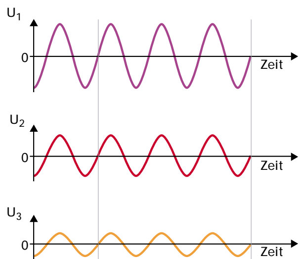
Spannungsamplituden in Abhängigkeit der Rotorstellung zur Empfangsspule (Beispiel einer Rotorstellung)
